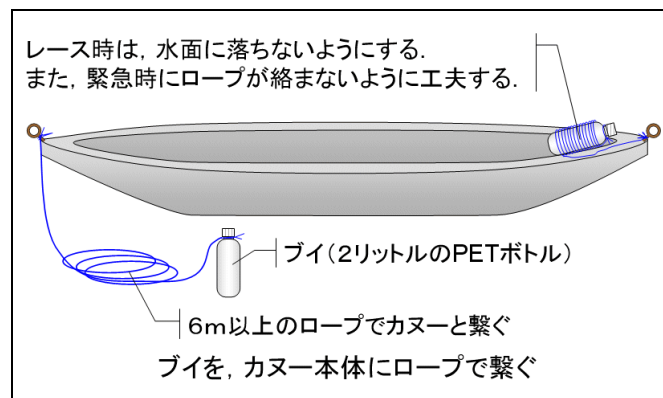
図-3 ブイ（目印用の浮き）の取付例
