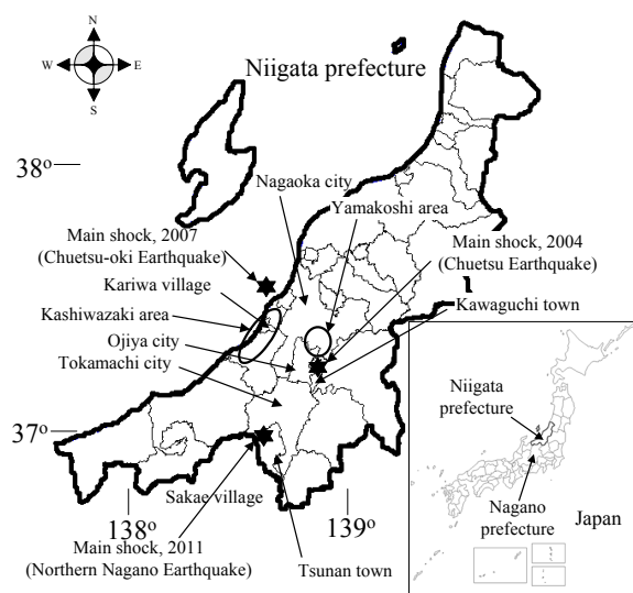
図3. 1-1 周辺で発生した地震の震央位置
