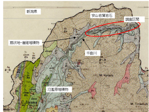
図2.1-1 長野県北部の表層地質図（表層地質図 1) を一部抜粋・加筆）
