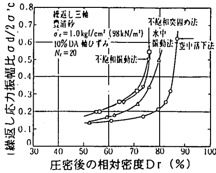
図-4.4.2 液状化強度比と相対密度の関係 7)
