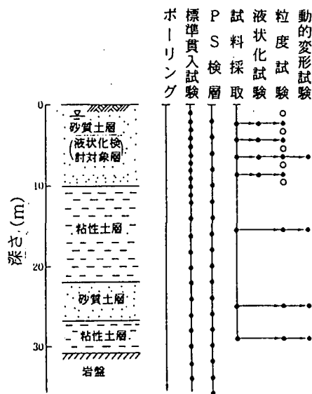
図-4.7.2 詳細な予測を行う場合の地質調査・試験項目及び実施数量の考え方 21)
