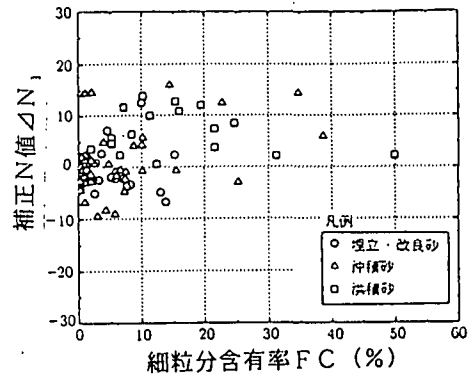
図-4.5.5 砂質土の補正項ΔN 1 と細粒分含有率FCの関係 10)
