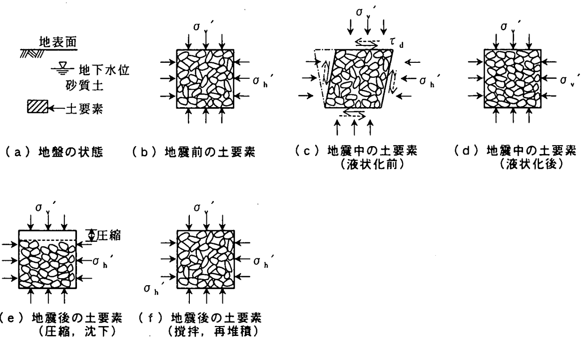
図-4.2.1 液状化発生のメカニズム 1)
