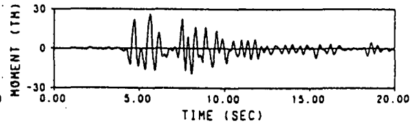
地下1階中柱下端 (A) の断面力
