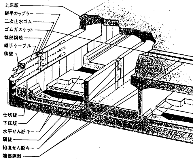
図-7.3.19 沈埋トンネルの可撓継手 27)
