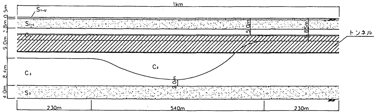
図-7.3.12 対象トンネルと地盤条件 2)
