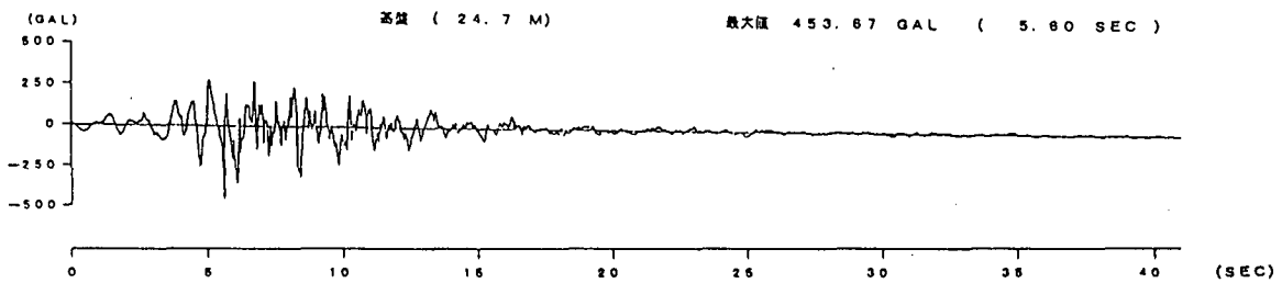
図-7.3.13 入力地震動 2)
