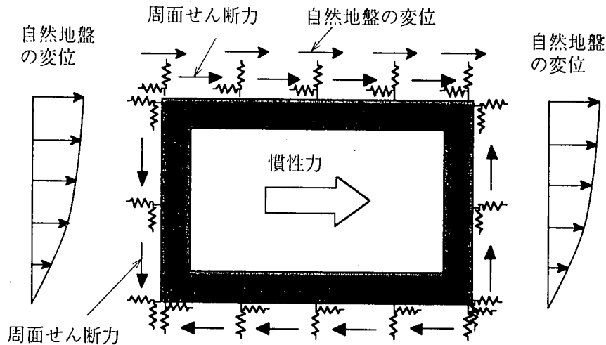
図-7.2.3 応答変位法の耐震計算モデル
