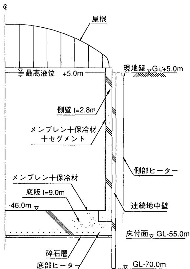
図-7.4.1 LNG地下タンクの一般構造図
