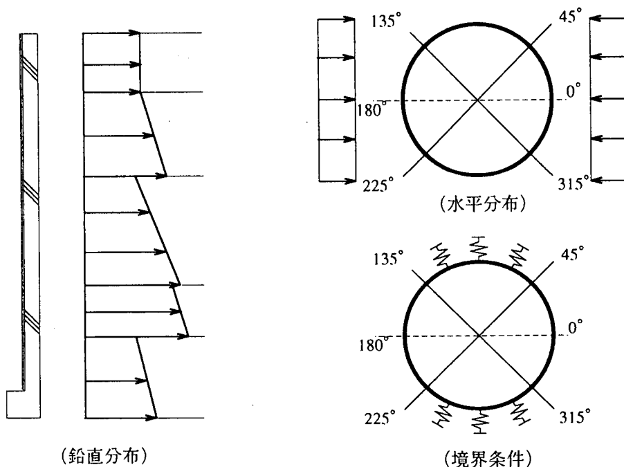
図-7.4.3 地震時土圧の荷重・境界条件
