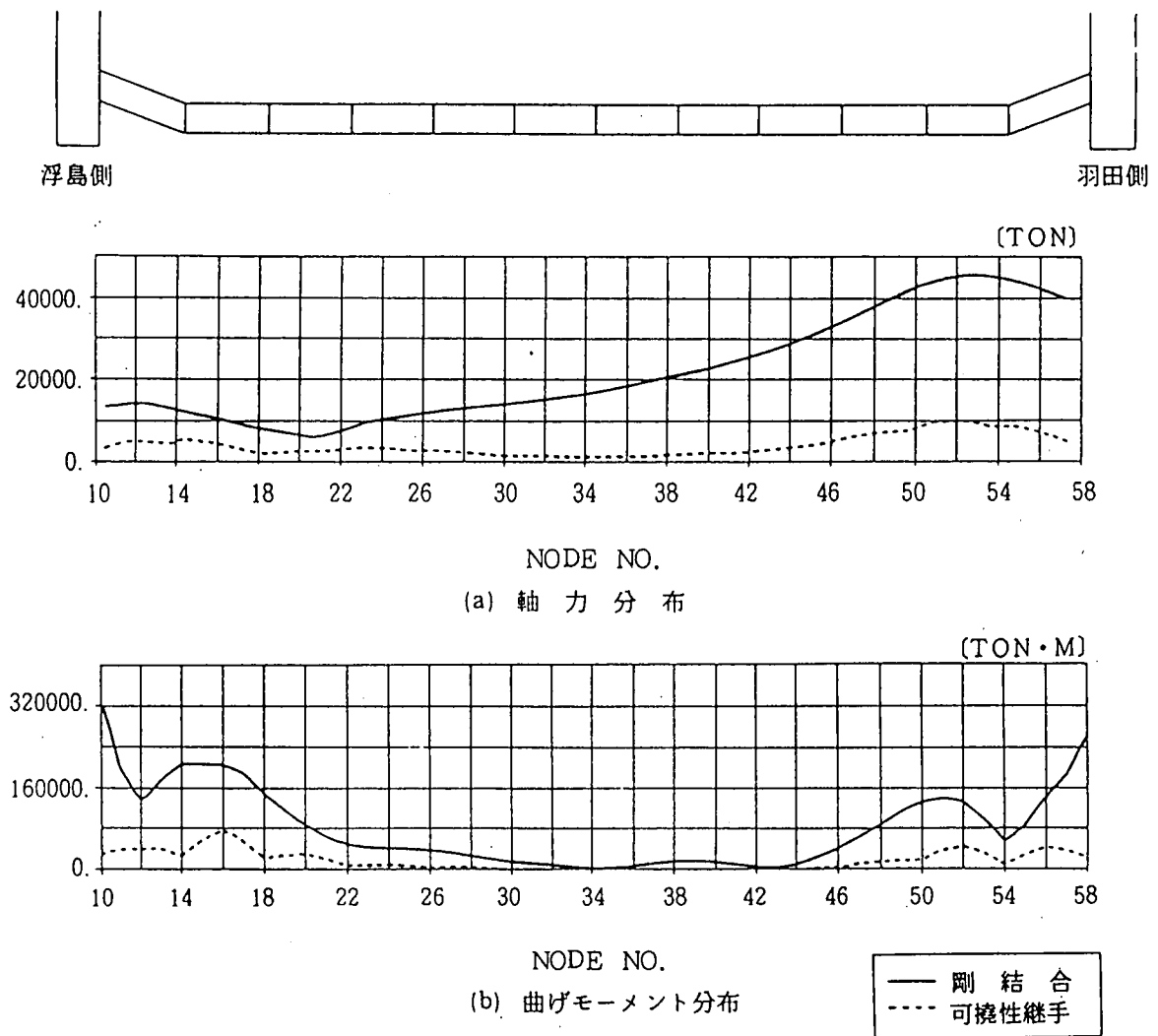
図-7.3.20 剛結合とした場合と可撓継手とした場合の断面力の比較 28)
