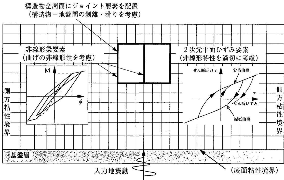
図-7.2.16 地盤-構造物の連成モデル
