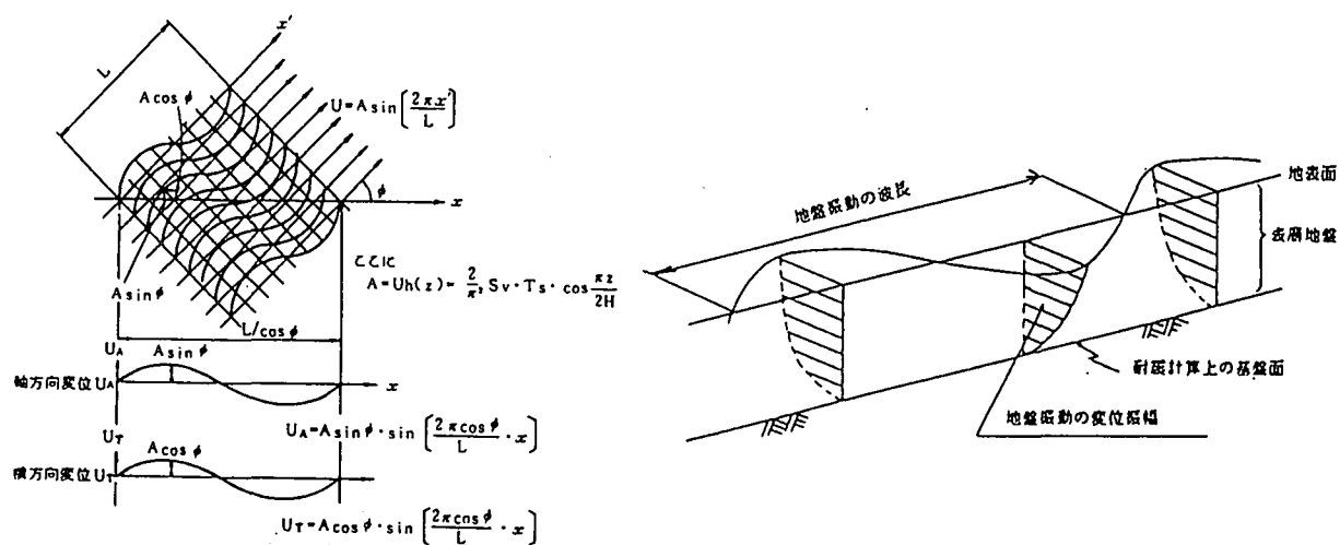
図-7.3.7 地盤変位分布の考え方 2,3, 2,4)
