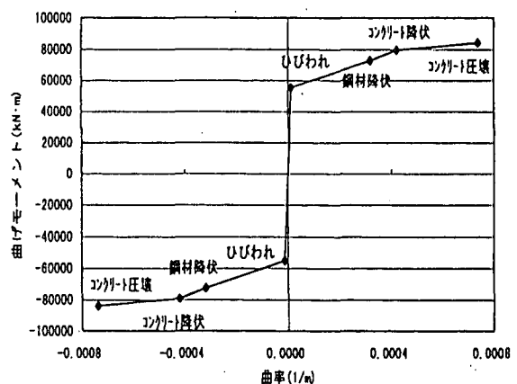
図-7.3.17 曲げモーメント～曲率の関係 22)
