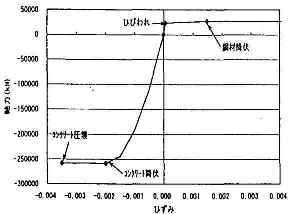
図-7.3.16 軸力～軸ひずみの関係 22)
