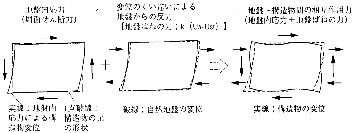
図-7.2.10 自然地盤による地震荷重の評価
