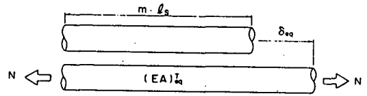
(b) 等価剛性梁モデル
