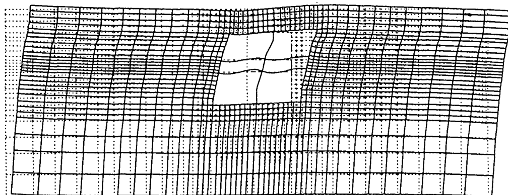
図-7.2.24 変形図 18)
