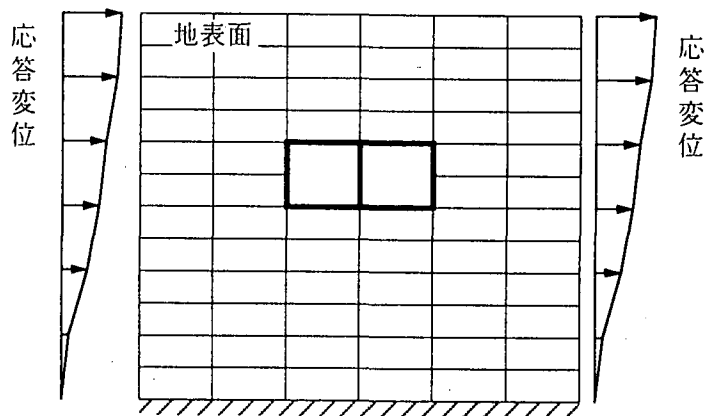
図-7.2.6 FEM応答変位法の解析モデル概念図
