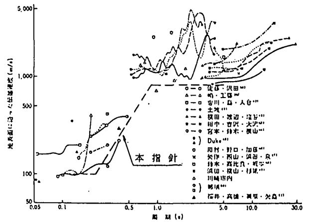
図-7.3.9 地震波の見かけの伝播速度 2,5)
