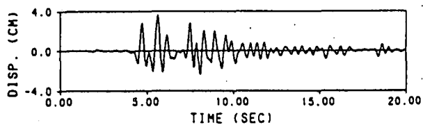
中柱のフロー間相対変位
