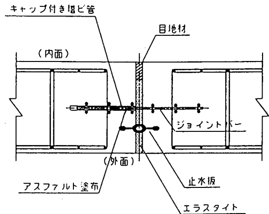
図-7.3.5 開削トンネルの伸縮目地 2,2)
