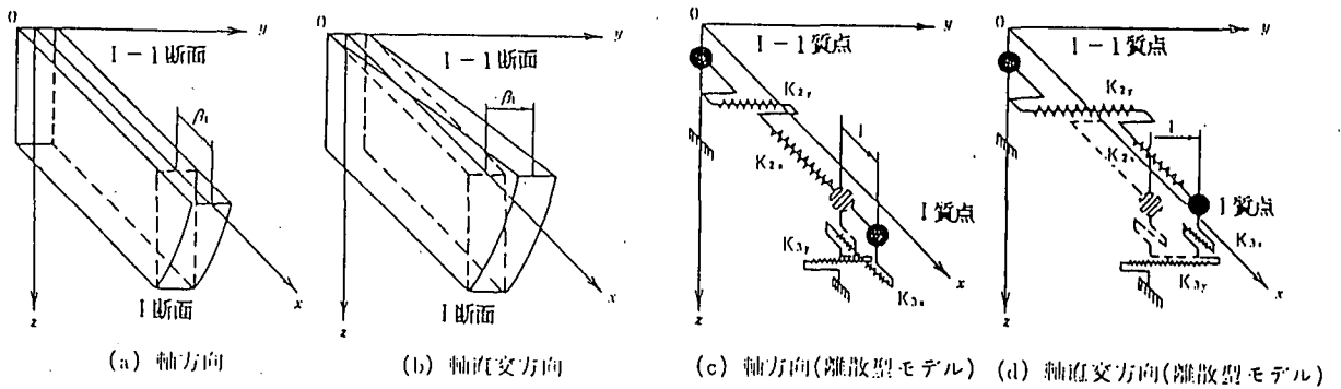
図-7.3.15 質点間バネの算定法 38)
