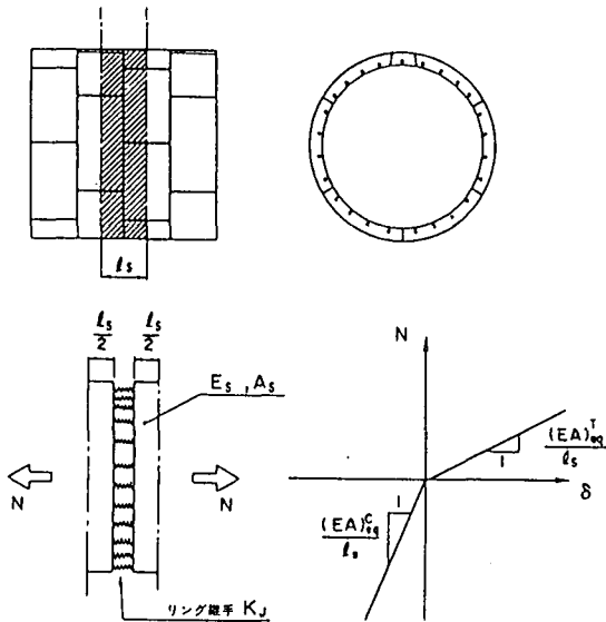
(c) 等価軸剛性
