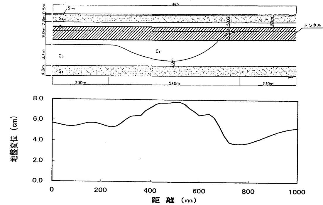
(a) 地盤の最大変位分布 [トンネル中心深さ]
