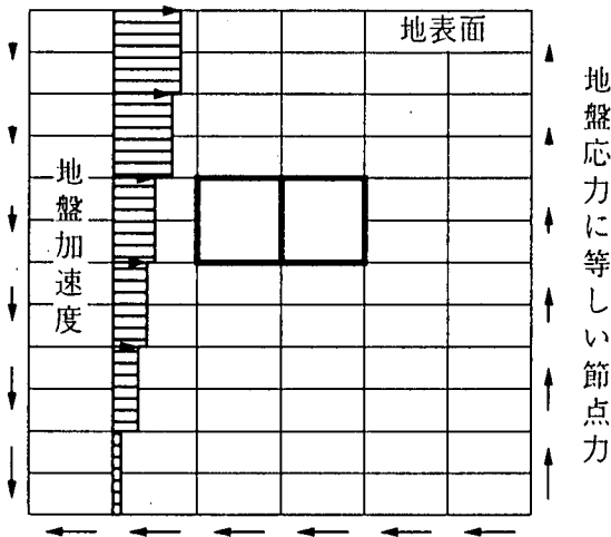
図-7.2.5 地盤応答法の解析モデル概念図
