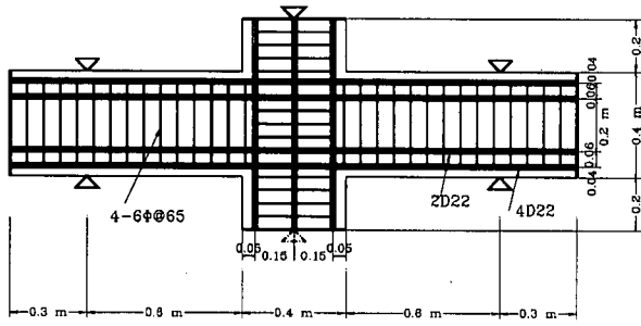
図-9 RC 構造の柱-梁接合部の交番載荷実験の供試体
