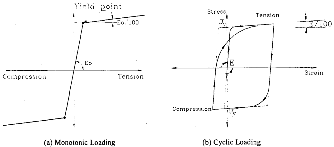
図-4 鉄筋の材料モデル
