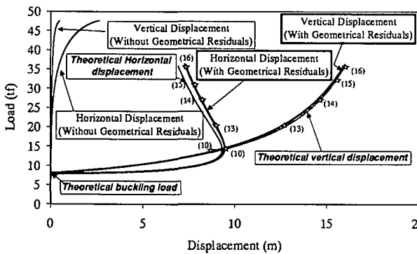
図-16 AEM 解析と理論解との比較
