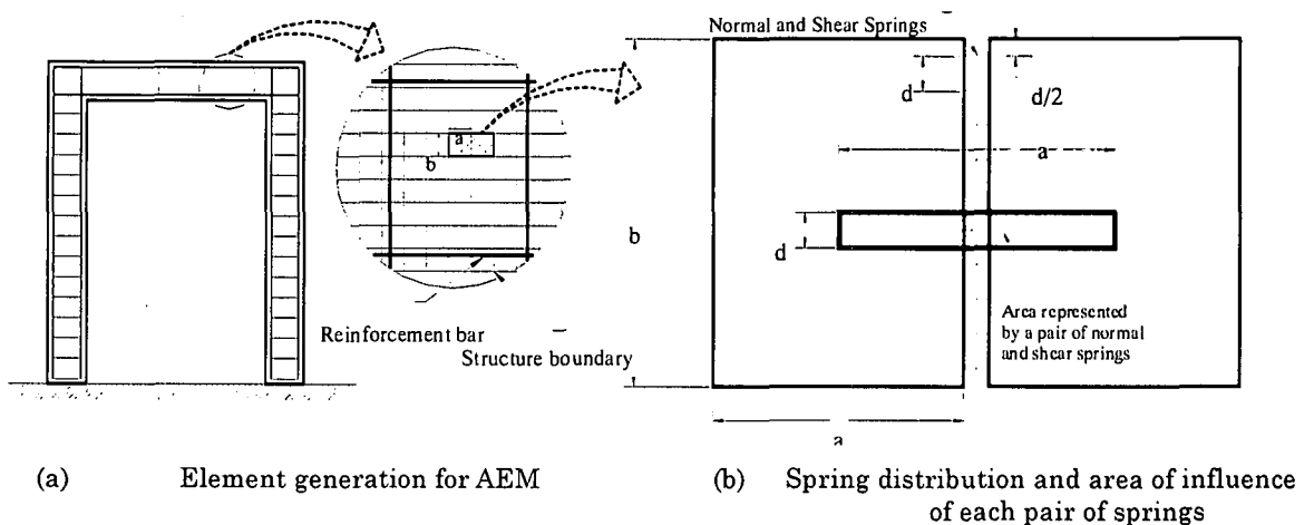
図-1 AEMにおける構造物のモデル化
