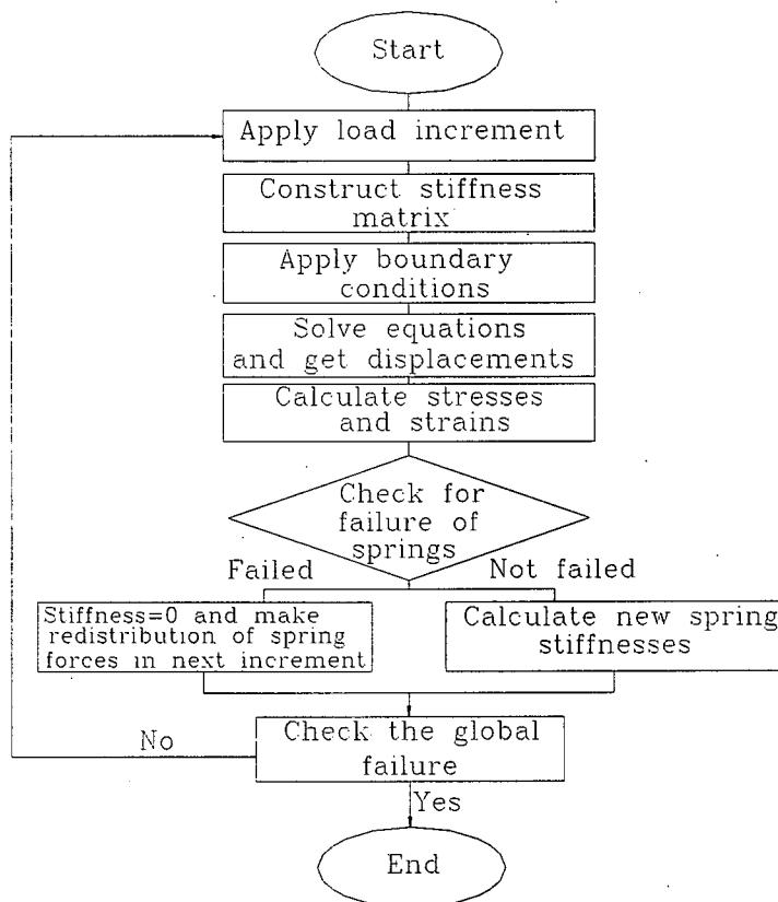
図-6 AEM 解析のフローチャート
