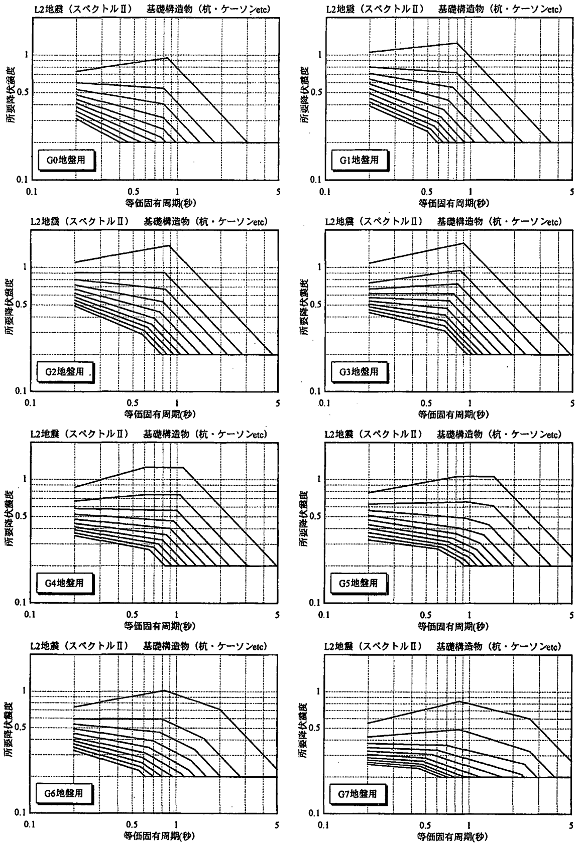
図-8.2.10 基礎構造物用の所要降伏震度スペクトルの例
