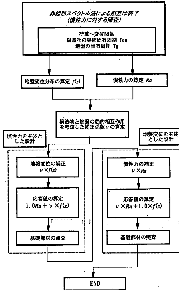
図-8.2.14 応答変位法により基礎構造物の応答値を算定するフロー
