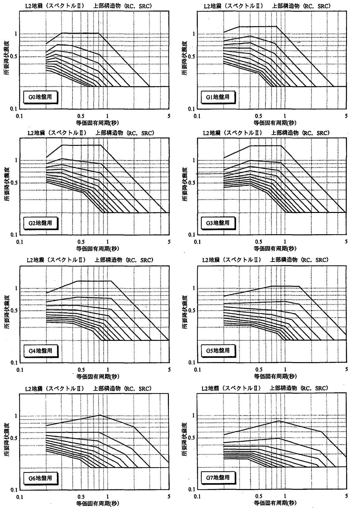
図-8.2.9 上部構造物用所要降伏震度スペクトルの例
