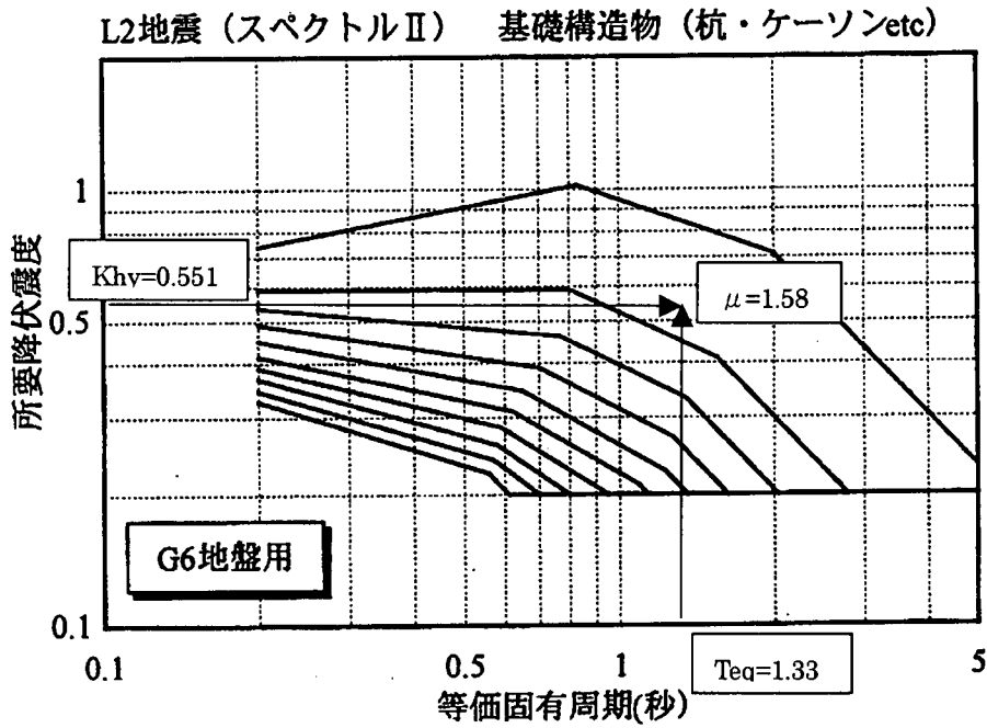
図-8.4.8 所要降伏震度スペクトルによる応答塑性率の算定
