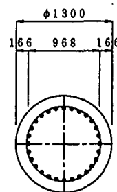
場所打ち杭（アースドリル杭）の断面形状
